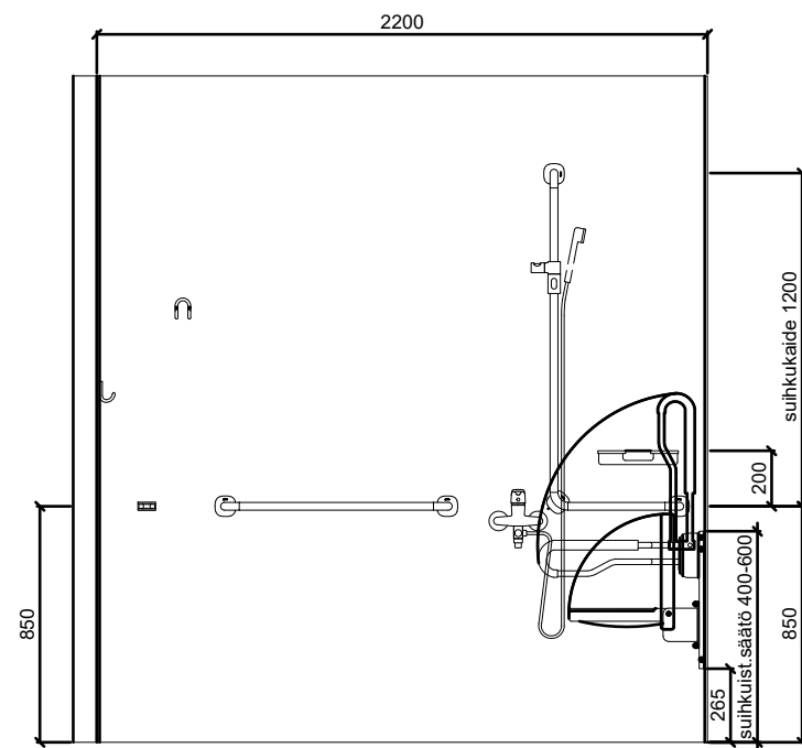
SEINÄKAAVIO C Gaius Original Classic 2XL W
