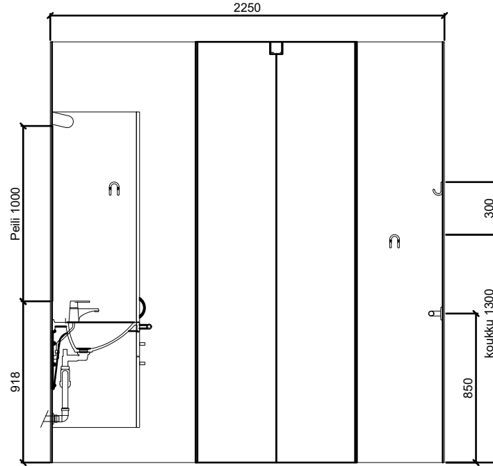
SEINÄKAAVIO B Gaius Original Classic 2XL W
