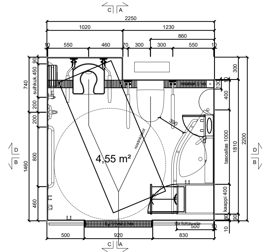
POHJAPIIRROS Gaius Original Classic 2XL W
