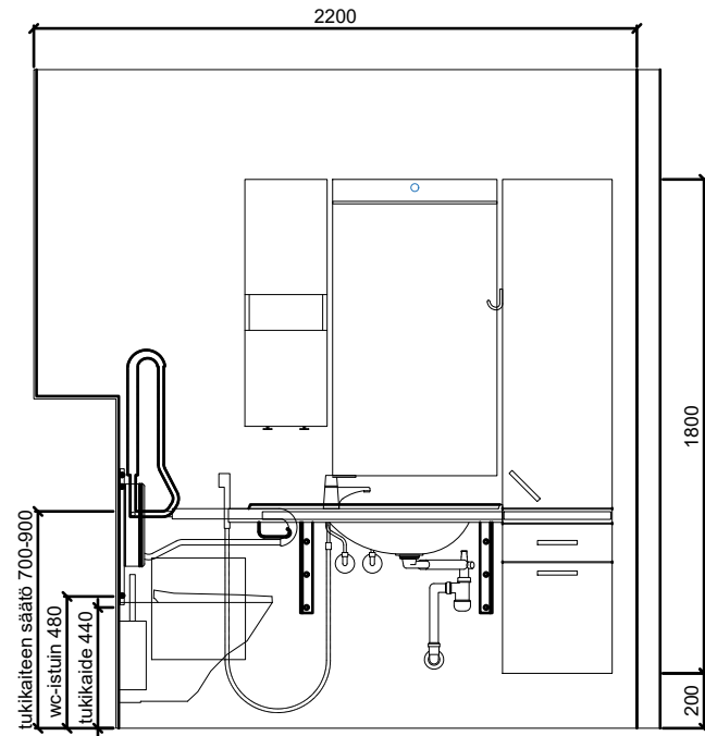
SEINÄKAAVIO A Gaius Original Classic 2XL W
