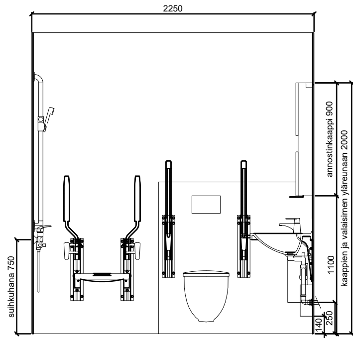
SEINÄKAAVIO D Gaius Original Classic 2XL W
