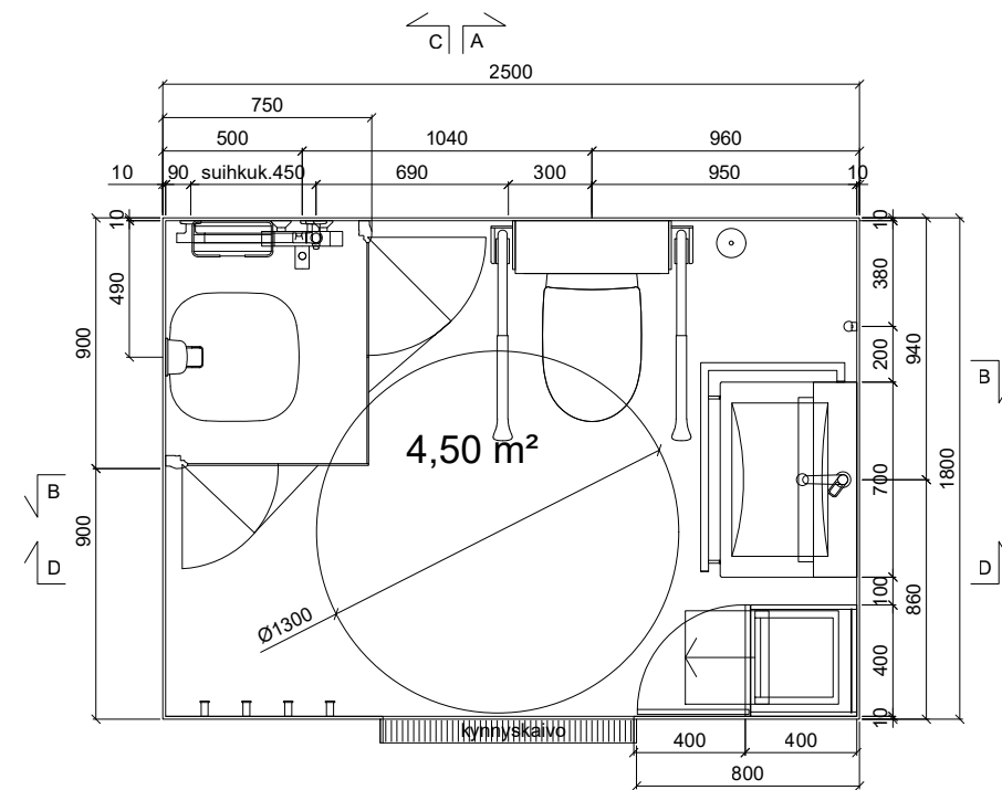
POHJAPIIRROS Gaius Life, DUO
