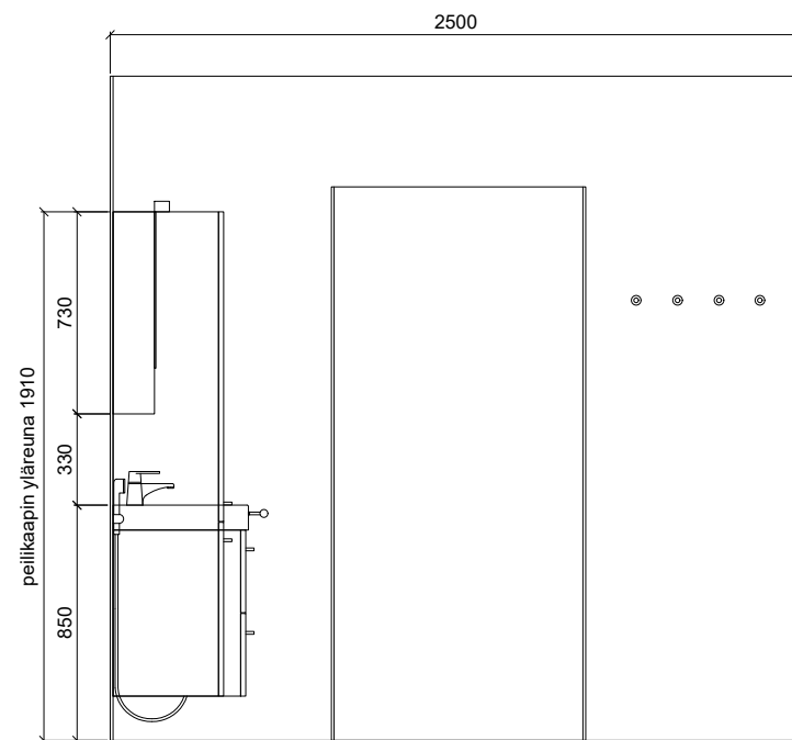
SEINÄKAAVIO B Gaius Life, DUO
