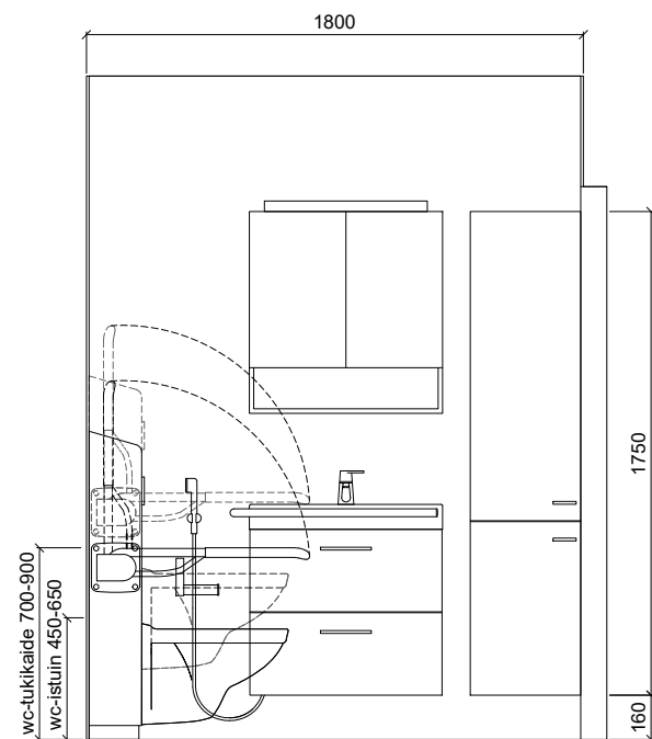
SEINÄKAAVIO A Gaius Life, DUO
