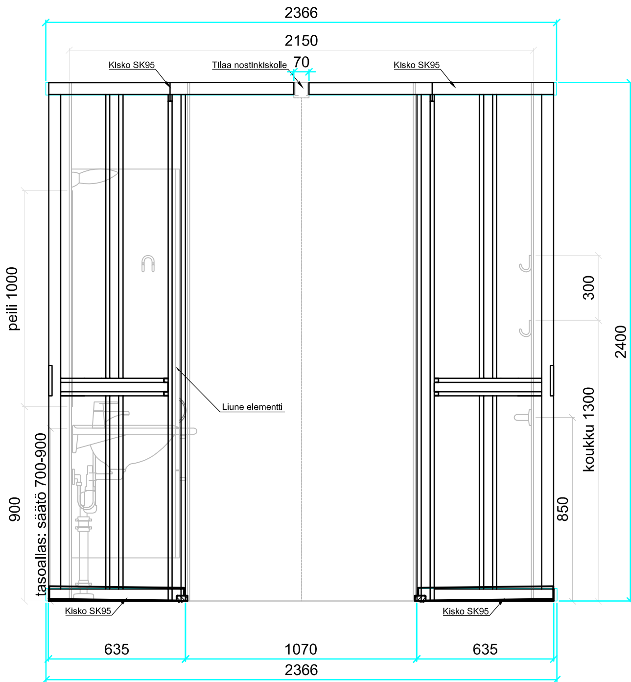
SEINÄKAAVIO B Gaius Original 2XL
