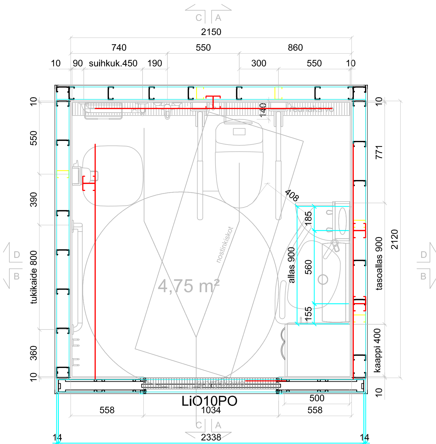
POHJAPIIRROS Gaius Original 2XL
