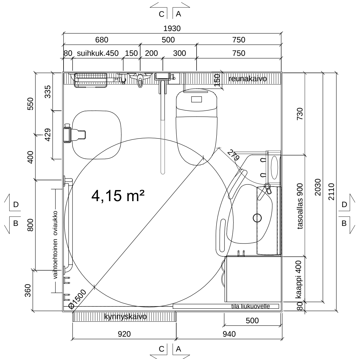
POHJAPIIRROS Gaius Original
