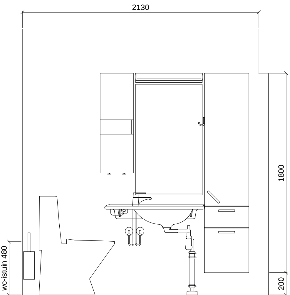
SEINÄKAAVIO A Gaius Original
