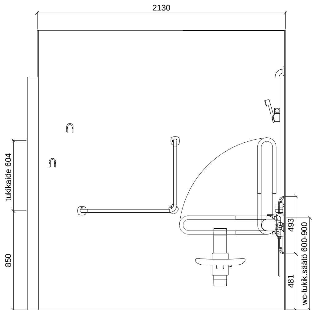
SEINÄKAAVIO C Gaius Original
