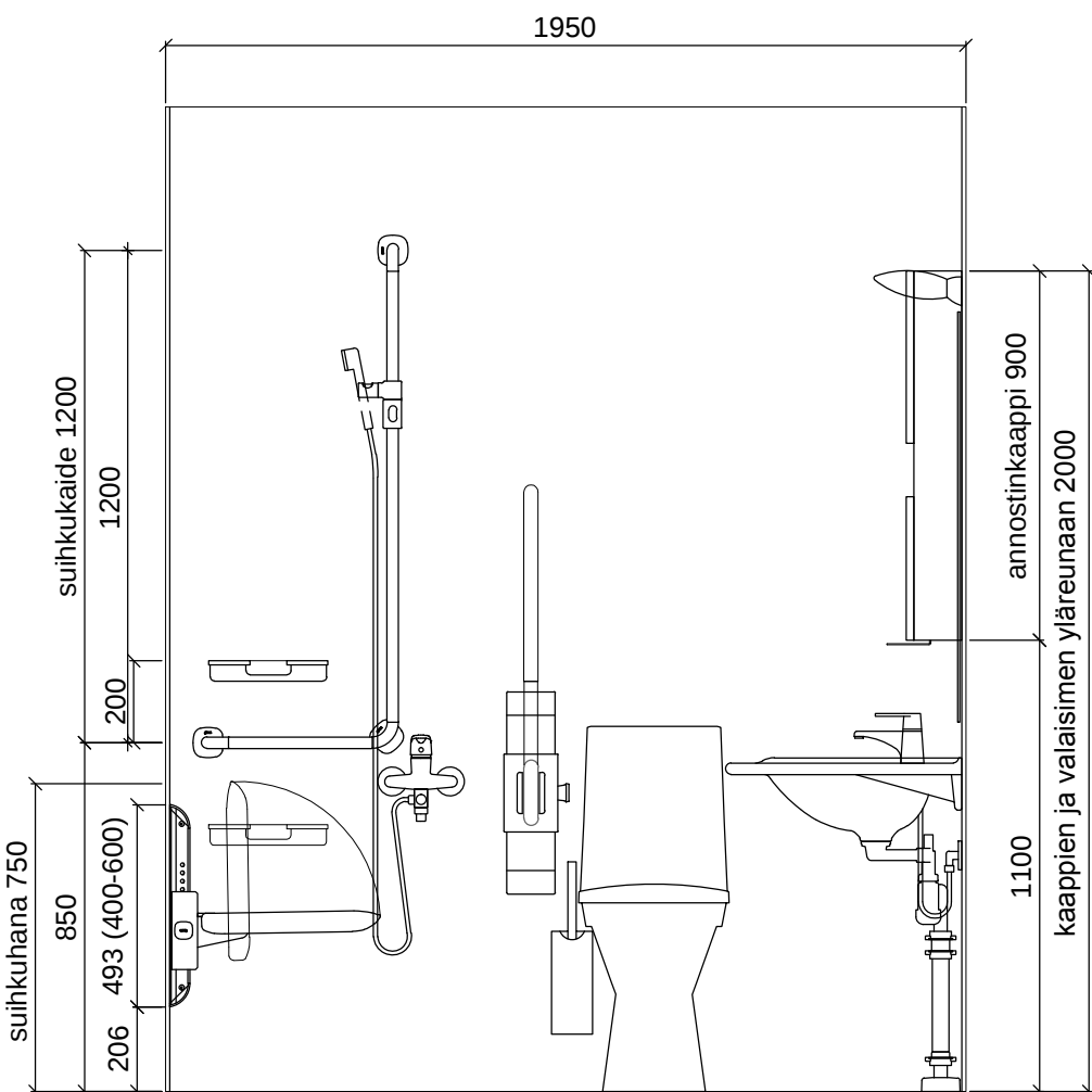
SEINÄKAAVIO D Gaius Original
