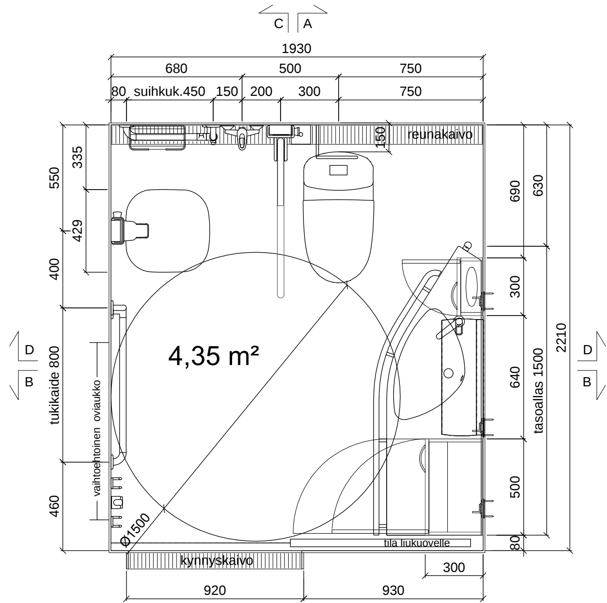
POHJAPIIRROS Gaius Original Plus
