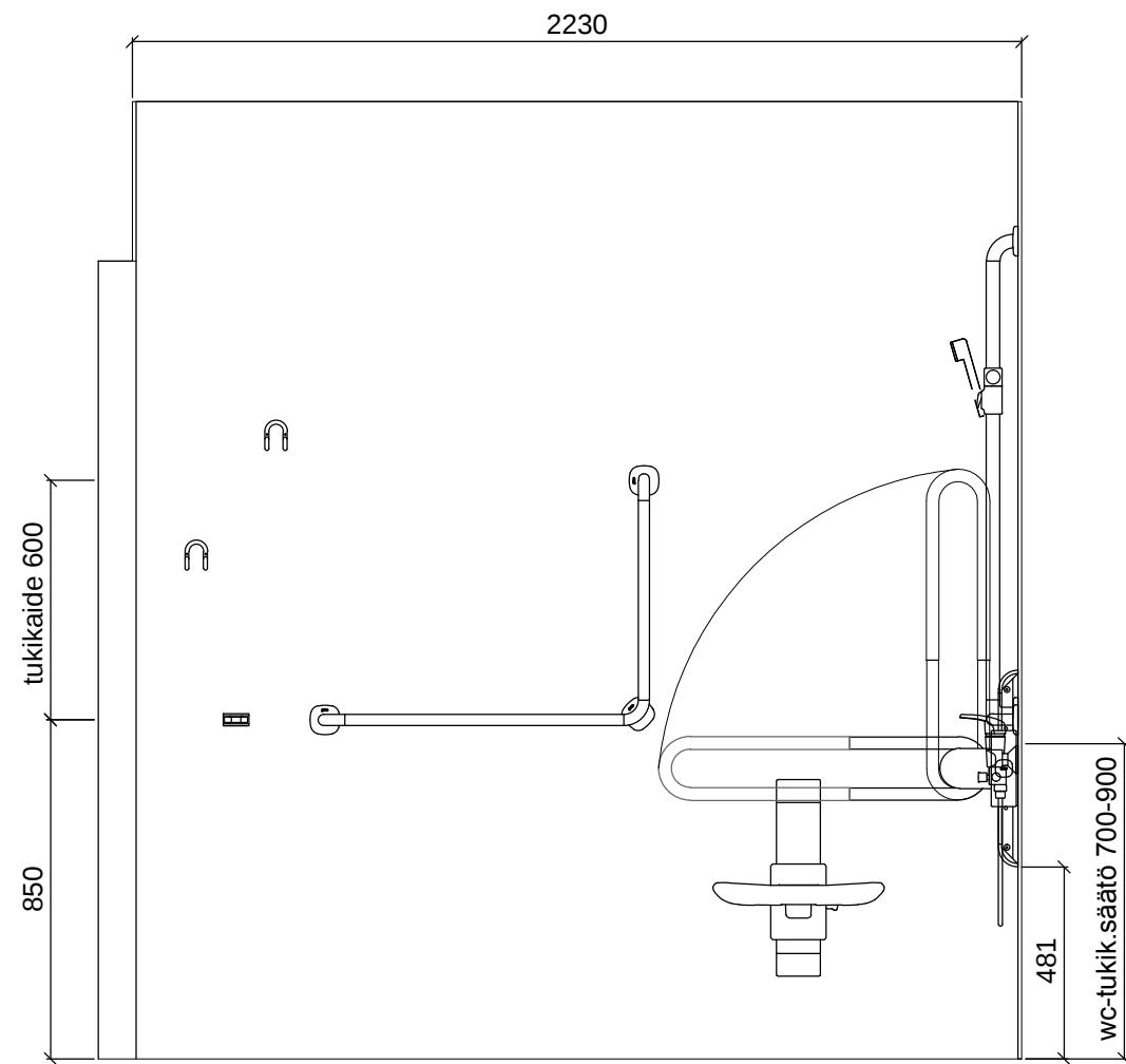
SEINÄKAAVIO C Gaius Original Plus
