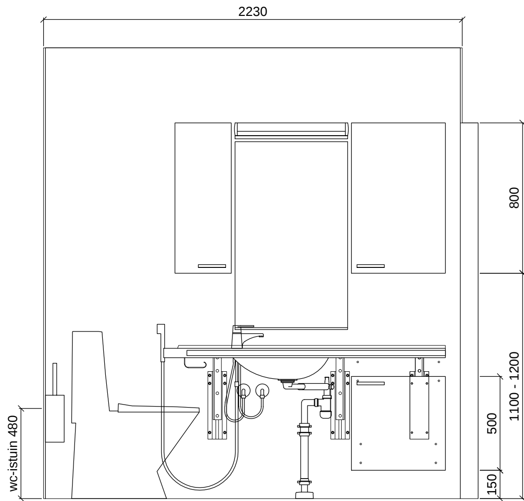
SEINÄKAAVIO A Gaius Original Plus
