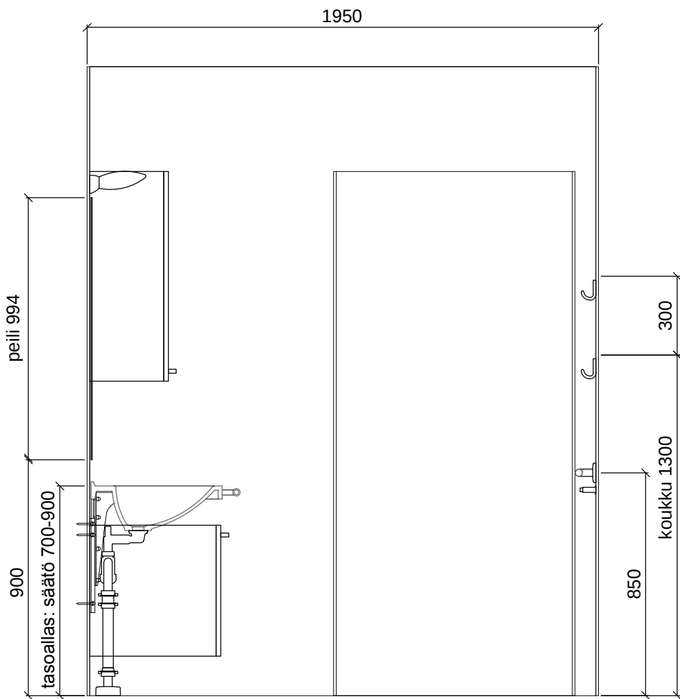
SEINÄKAAVIO B Gaius Original Plus
