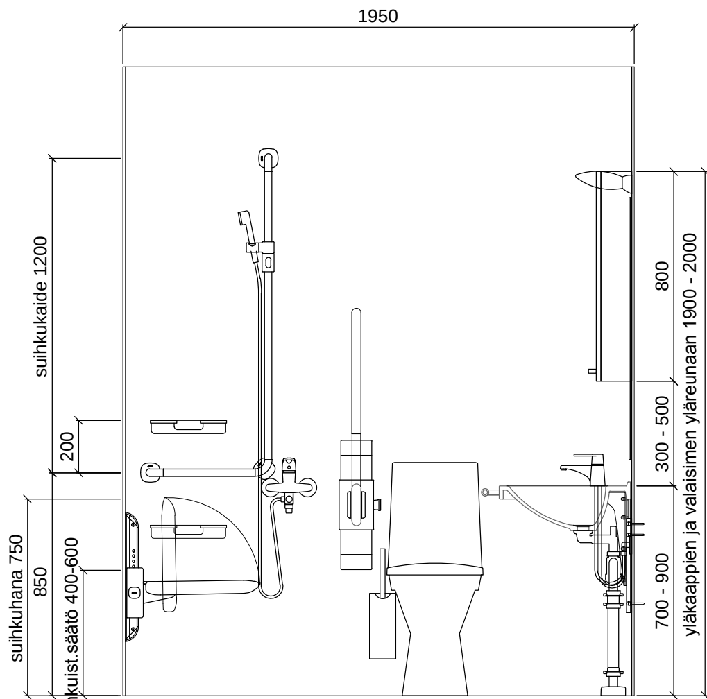
SEINÄKAAVIO D Gaius Original Plus
