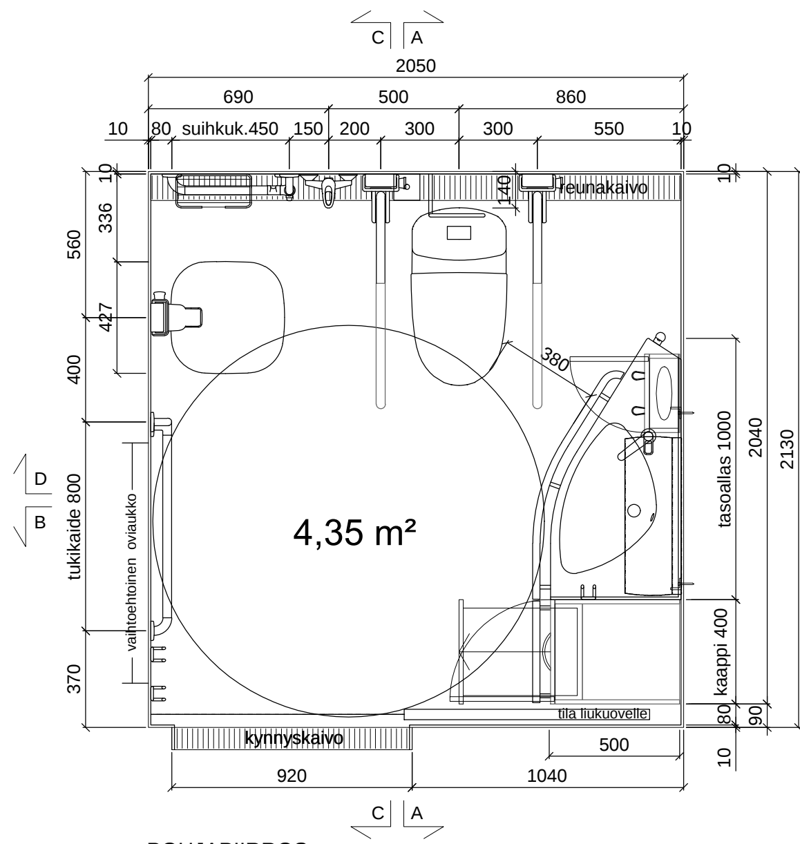
POHJAPIIRROS Gaius Original XL
