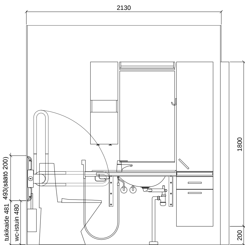
SEINÄKAAVIO A Gaius Original XL
