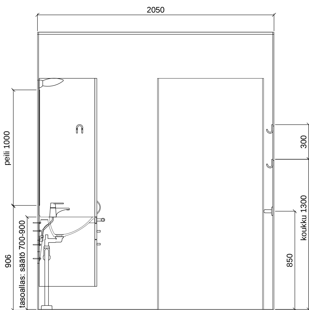
SEINÄKAAVIO B Gaius Original XL
