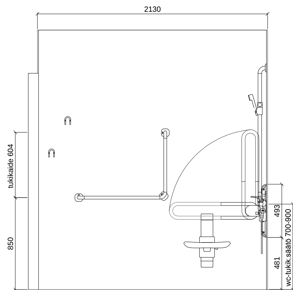
SEINÄKAAVIO C Gaius Original XL
