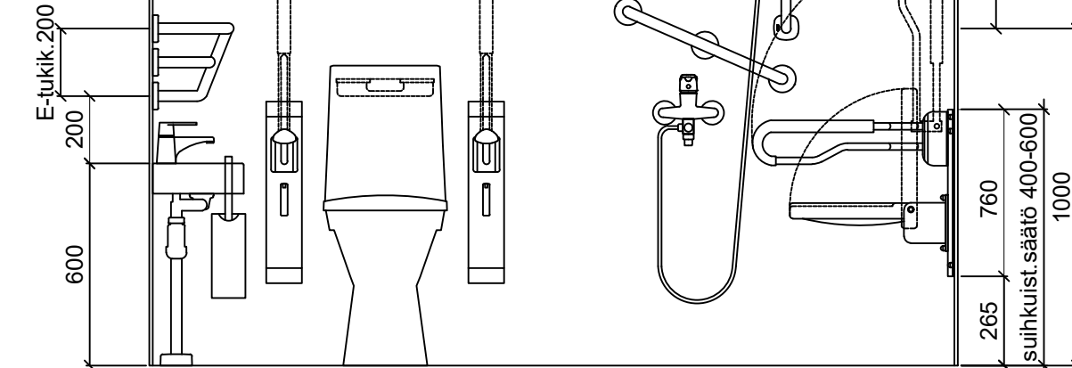
SEINÄKAAVIO C Gaius Hospital 2XL
