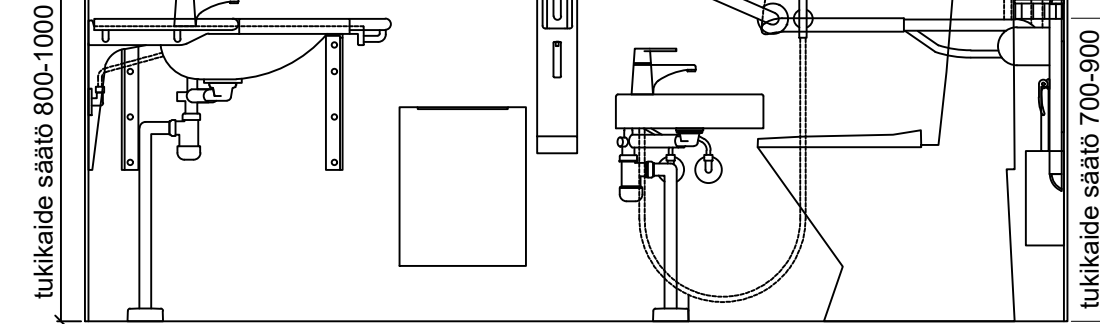
SEINÄKAAVIO B Gaius Hospital 2XL
