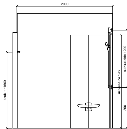
SEINÄKAAVIO C Gaius Life XL
