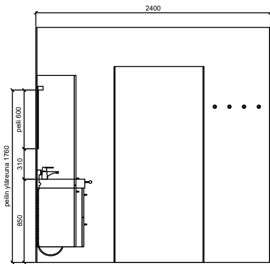
SEINÄKAAVIO B Gaius Life XL
