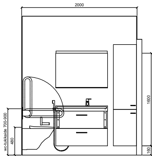
SEINÄKAAVIO A Gaius Life XL
