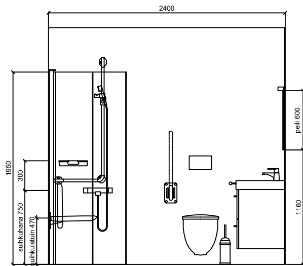
SEINÄKAAVIO D Gaius Life XL
