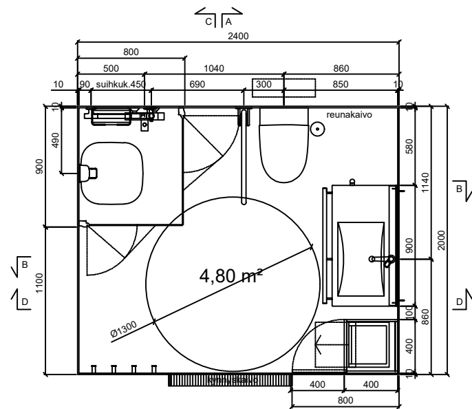
POHJAPIIRROS Gaius Life XL
