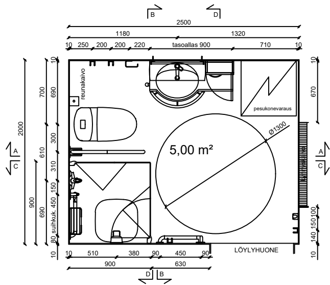
POHJAPIIRROS Senior XL
