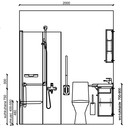
SEINÄKAAVIO D Senior XL
