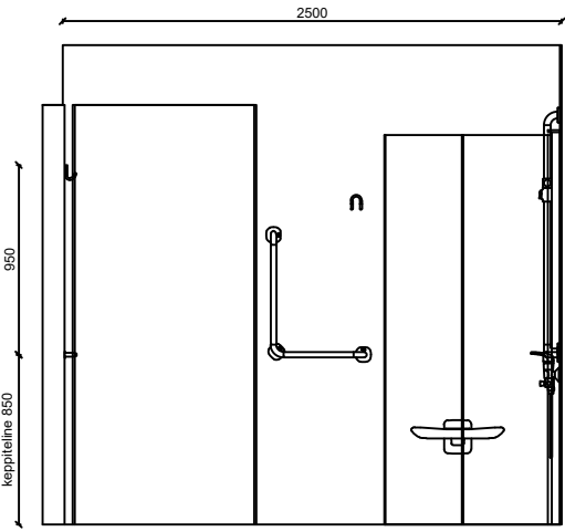
SEINÄKAAVIO C Senior XL
