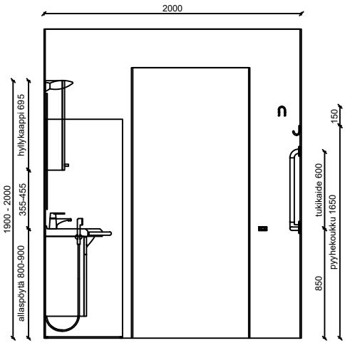
SEINÄKAAVIO B Senior XL
