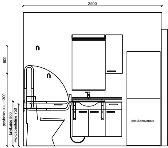
SEINÄKAAVIO A Senior XL
