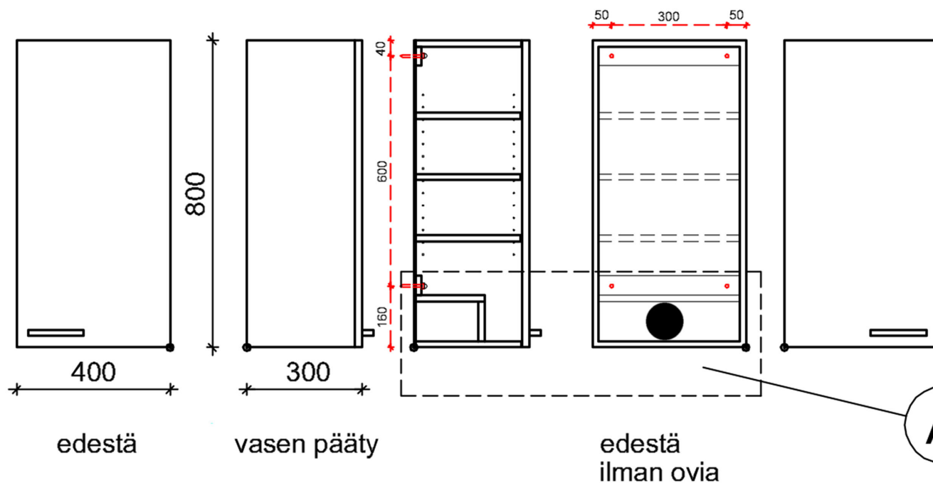
pystyleikkaus
