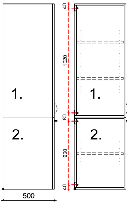
vasen pääty
