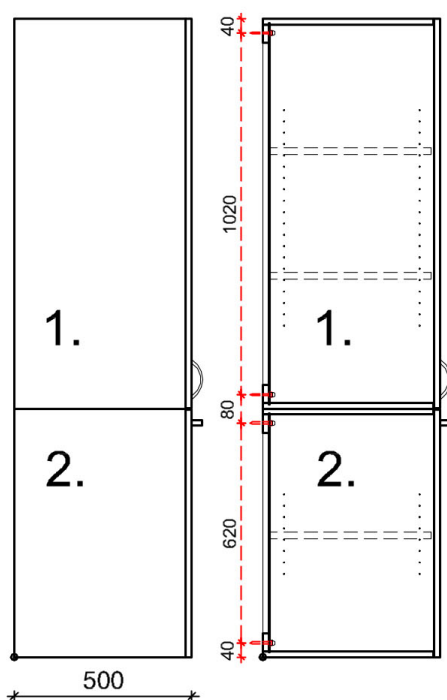
vasen pääty
