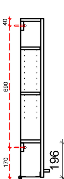
pystyleikkaus
