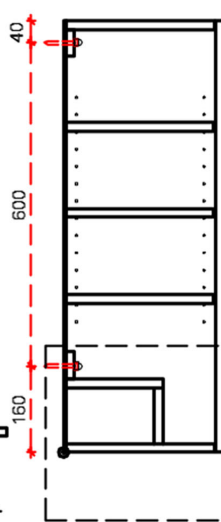
pystyleikkaus
