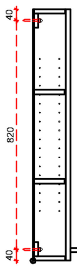
pystyleikkaus
