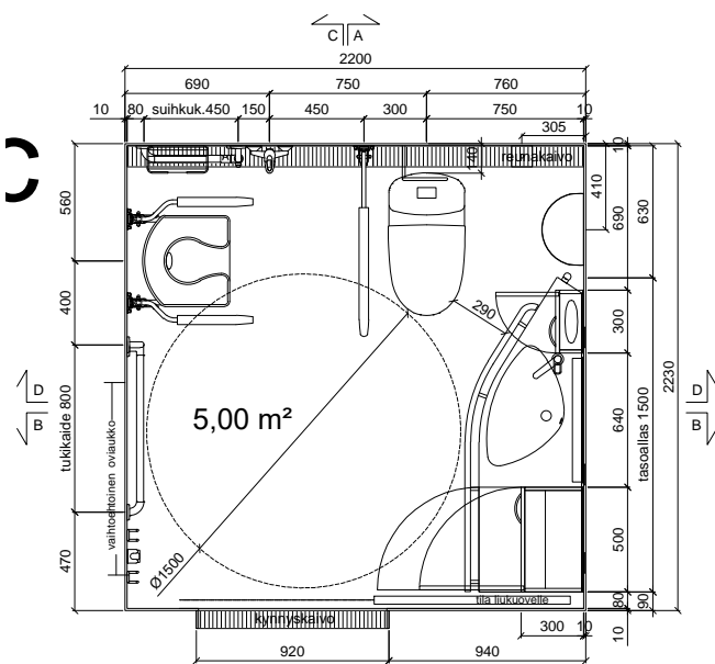
POHJAPIIRROS Gaius Original Classic Plus 1500
