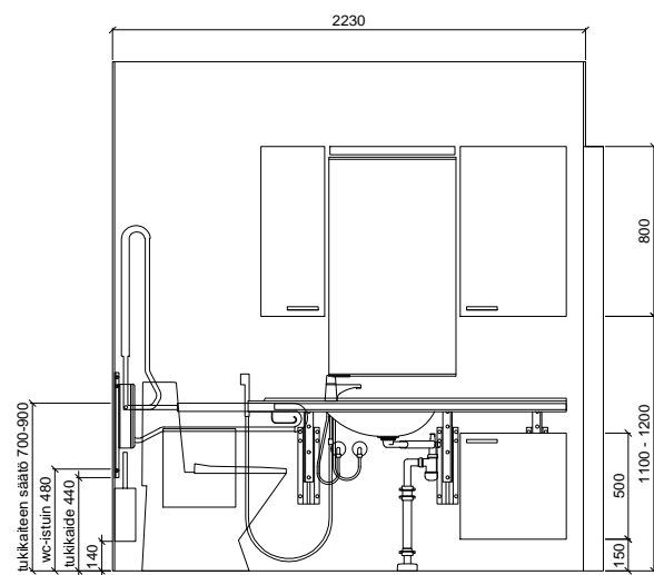
SEINÄKAAVIO A Gaius Original Classic Plus 1500
