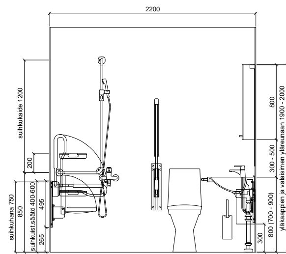
SEINÄKAAVIO D Gaius Original Classic Plus 1500
