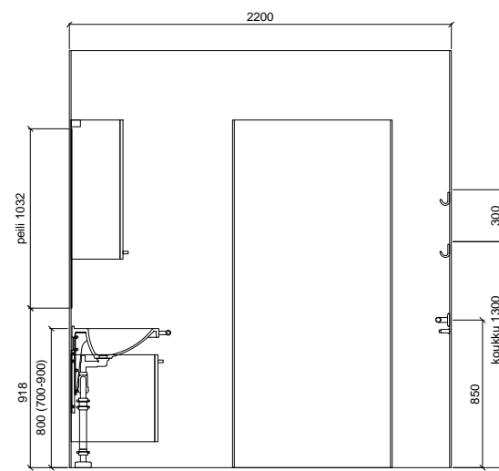
SEINÄKAAVIO B Gaius Original Classic Plus 1500
