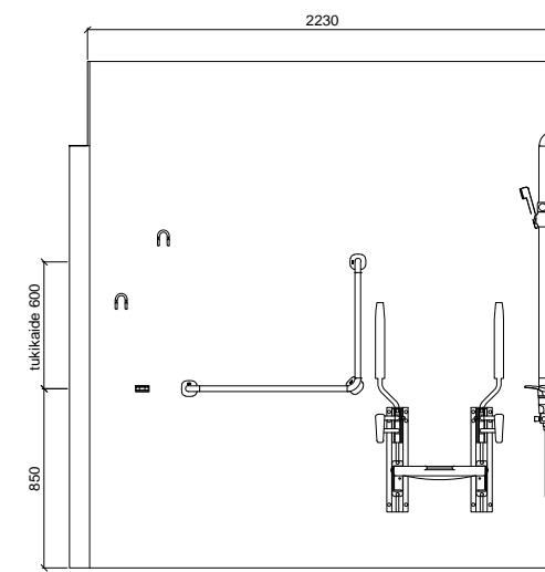
SEINÄKAAVIO C Gaius Original Classic Plus 1500
