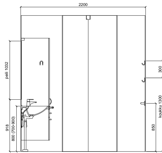
SEINÄKAAVIO B Gaius Original Classic 2XL
