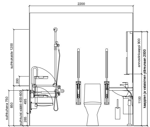
SEINÄKAAVIO D Gaius Original Classic 2XL
