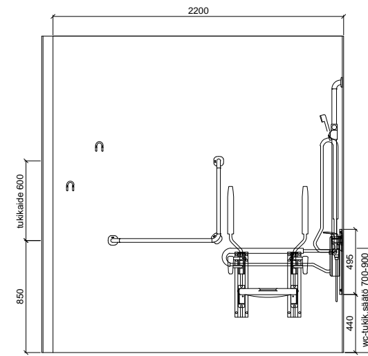
SEINÄKAAVIO C Gaius Original Classic 2XL
