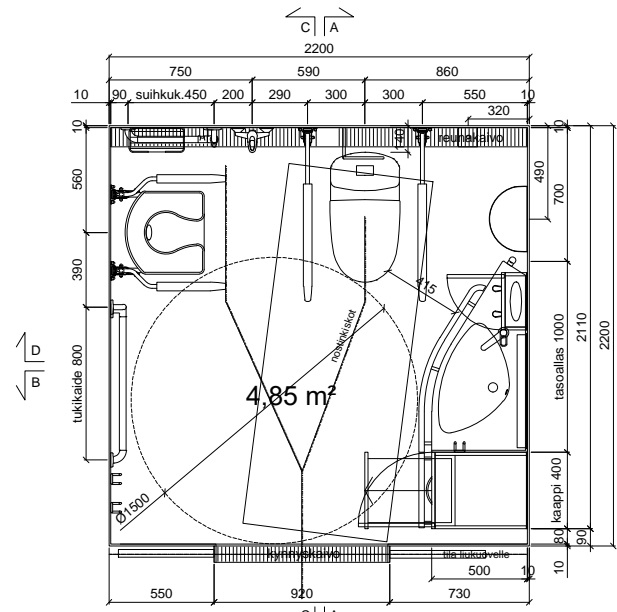
POHJAPIIRROS Gaius Original Classic 2XL
