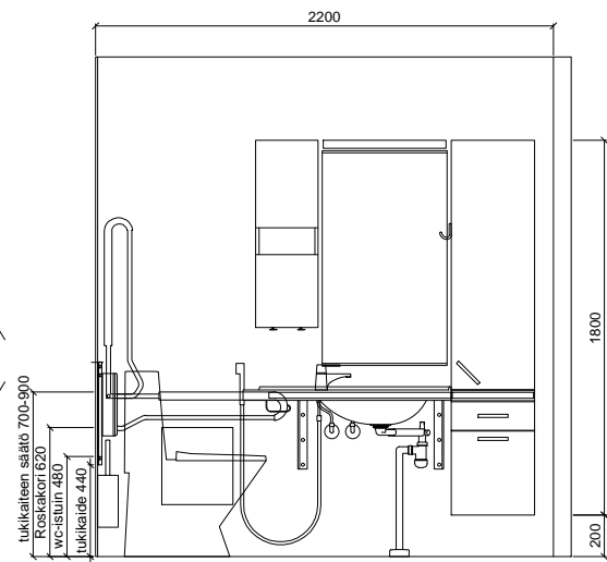
SEINÄKAAVIO A Gaius Original Classic 2XL
