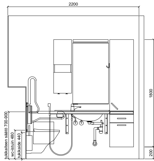
SEINÄKAAVIO A Gaius Original Classic 2XL W
