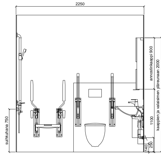
SEINÄKAAVIO D Gaius Original Classic 2XL W
