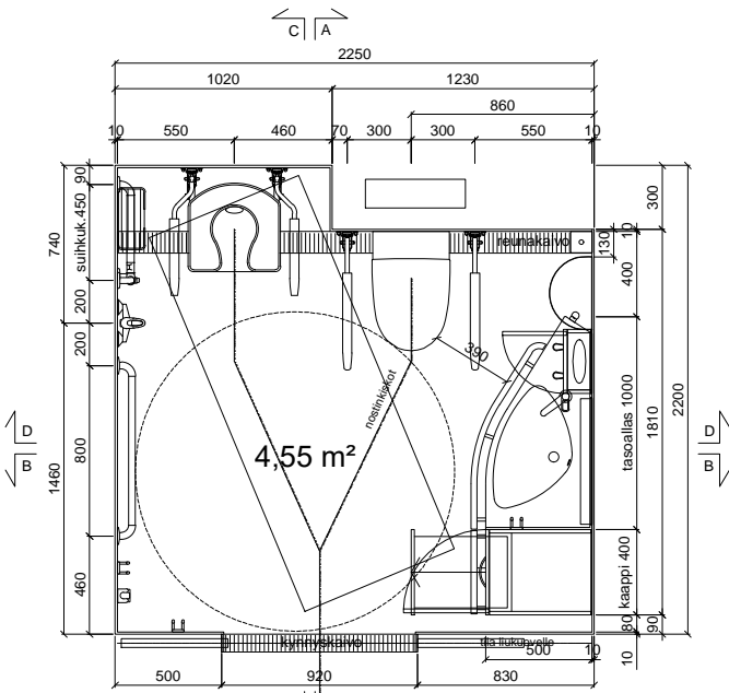
POHJAPIIRROS Gaius Original Classic 2XL W
