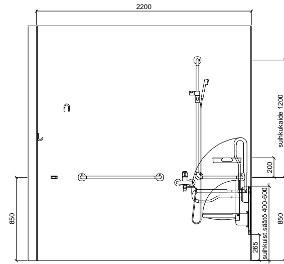
SEINÄKAAVIO C Gaius Original Classic 2XL W
