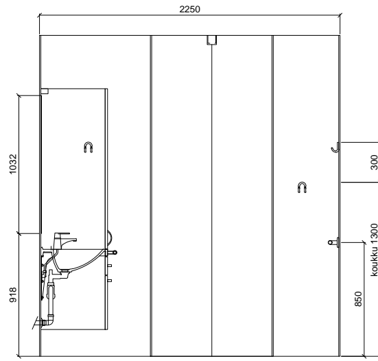
SEINÄKAAVIO B Gaius Original Classic 2XL W
