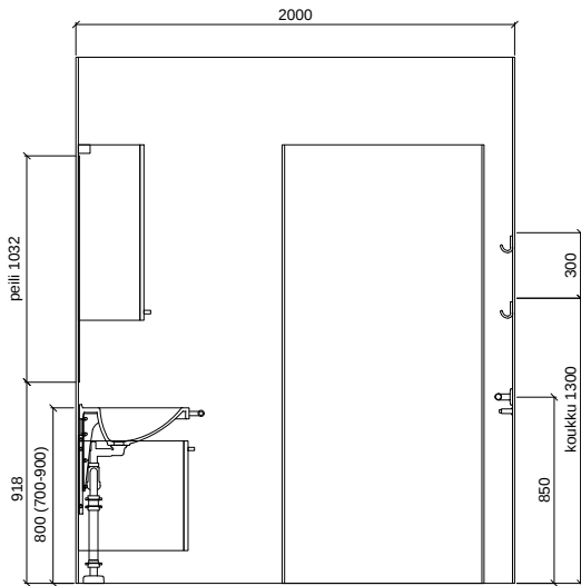
SEINÄKAAVIO B Gaius Original Classic Plus
