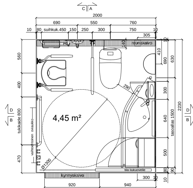
POHJAPIIRROS Gaius Original Classic Plus
