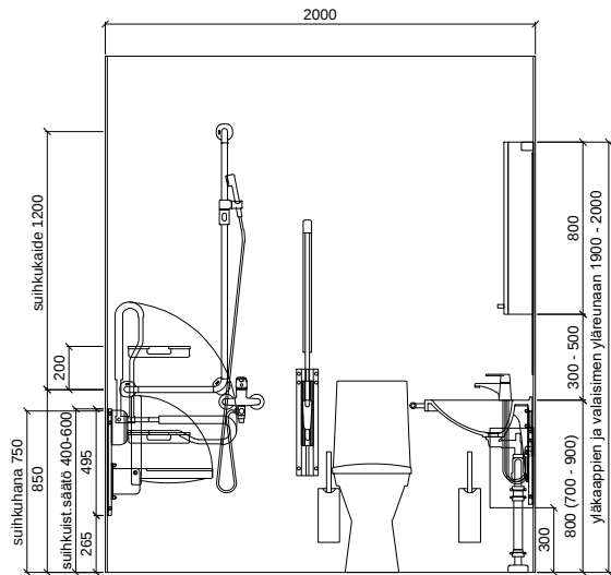
SEINÄKAAVIO D Gaius Original Classic Plus
