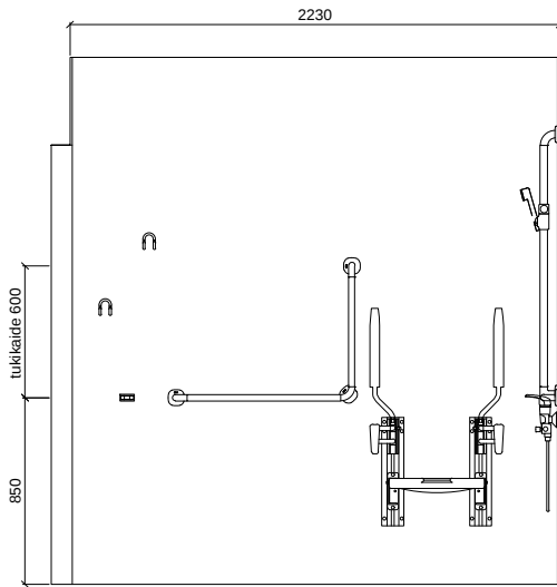
SEINÄKAAVIO C Gaius Original Classic Plus
