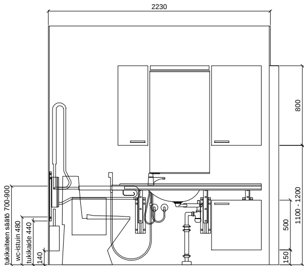
SEINÄKAAVIO A Gaius Original Classic Plus
