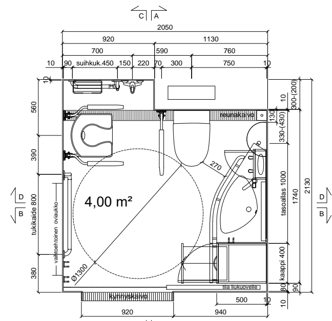
POHJAPIIRROS Gaius Original Classic W
