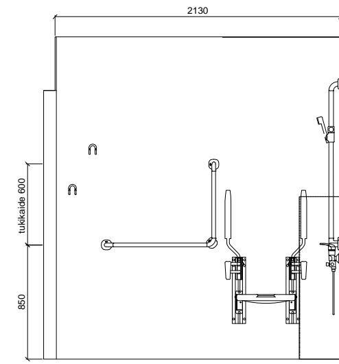
SEINÄKAAVIO C Gaius Original Classic W
