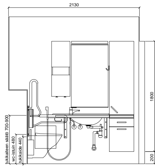
SEINÄKAAVIO A Gaius Original Classic W
