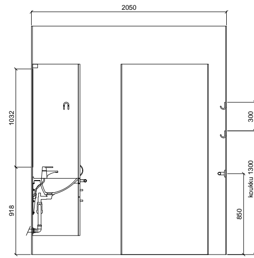
SEINÄKAAVIO B Gaius Original Classic W
