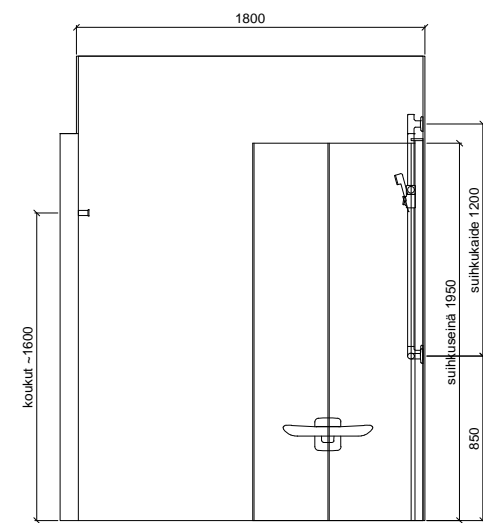
SEINÄKAAVIO C Gaius Life
