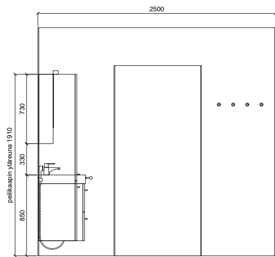
SEINÄKAAVIO B Gaius Life
