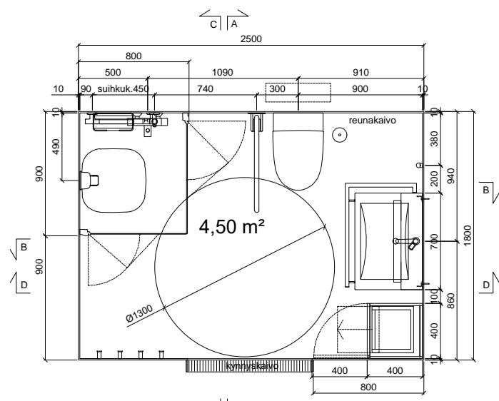
POHJAPIIRROS Gaius Life
