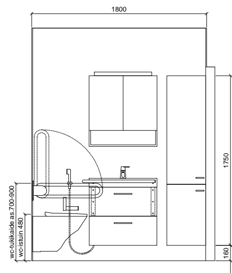
SEINÄKAAVIO A Gaius Life
