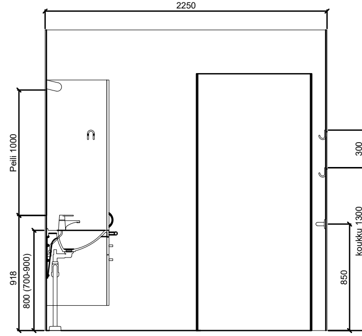
SEINÄKAAVIO B Gaius Original Classic XL
