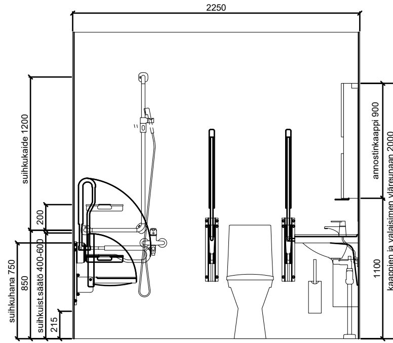
SEINÄKAAVIO D Gaius Original Classic XL
