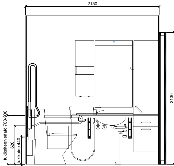
SEINÄKAAVIO A Gaius Original Classic XL
