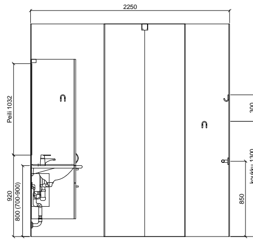
SEINÄKAAVIO B Gaius Original Sense 2XL W
