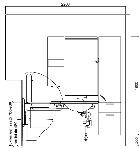
SEINÄKAAVIO A Gaius Original Sense 2XL W
