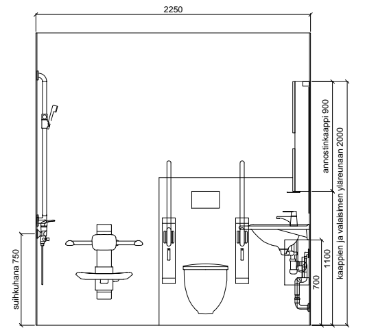
SEINÄKAAVIO D Gaius Original Sense 2XL W
