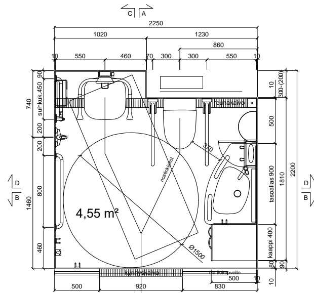
POHJAPIIRROS Gaius Original Sense 2XL W
