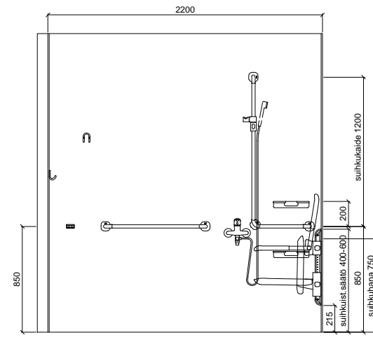
SEINÄKAAVIO C Gaius Original Sense 2XL W
