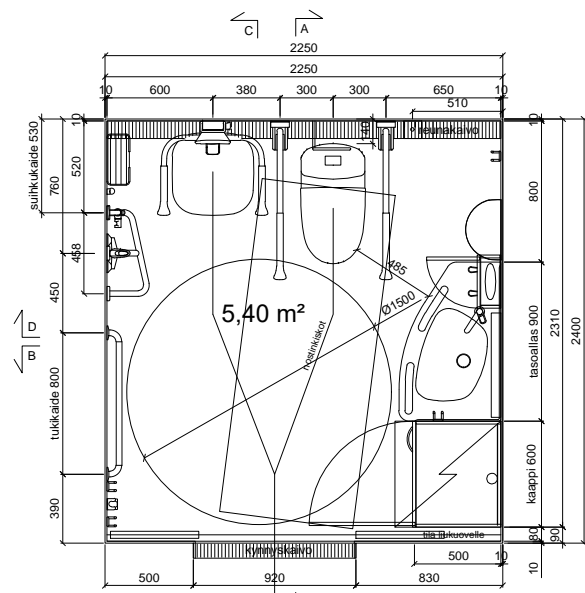
POHJAPIIRROS Gaius Original Sense 3XL
