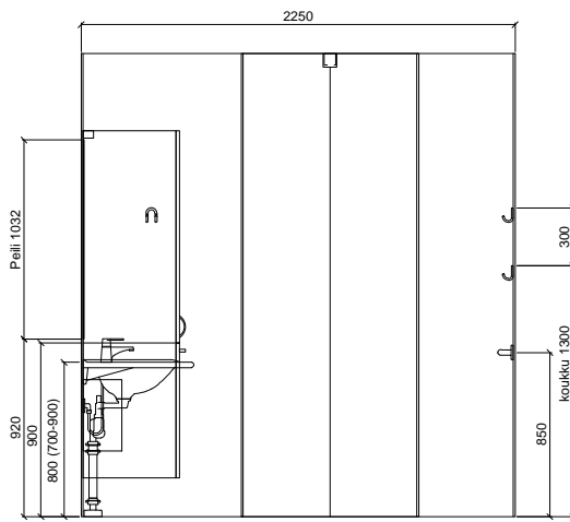
SEINÄKAAVIO B Gaius Original Sense 3XL
