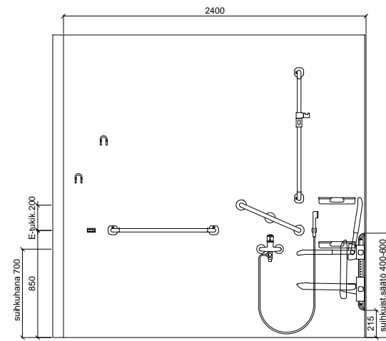
SEINÄKAAVIO C Gaius Original Sense 3XL
