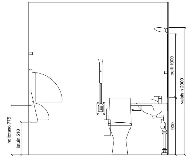
SEINÄKAAVIO H
