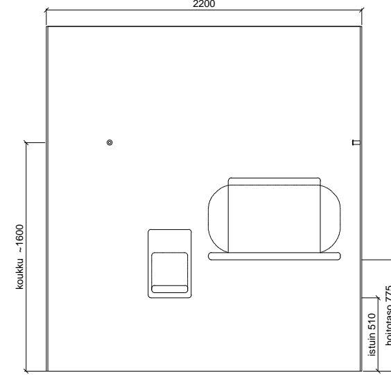
SEINÄKAAVIO G
