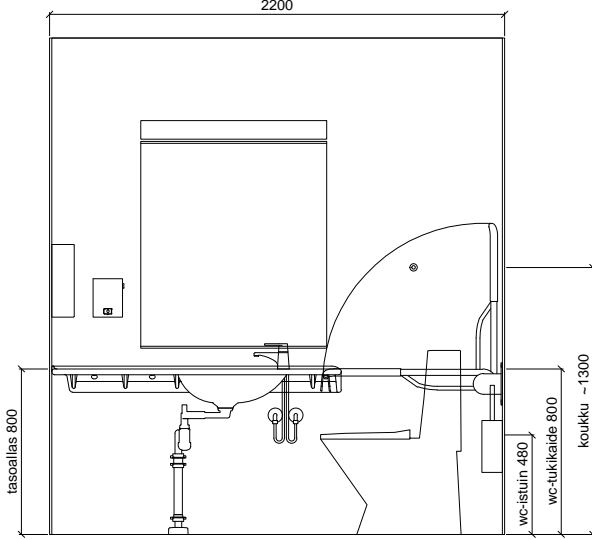
SEINÄKAAVIO E
