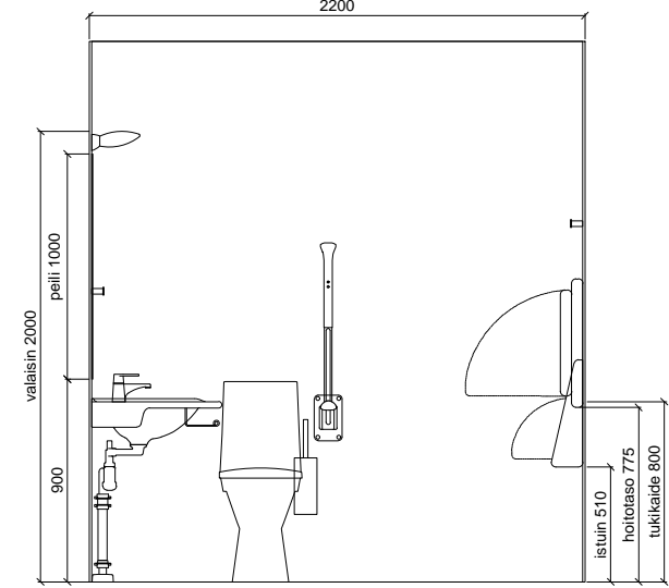
SEINÄKAAVIO H
