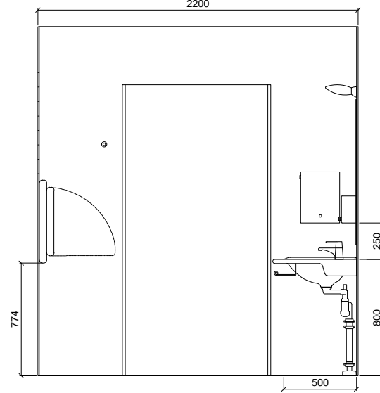
SEINÄKAAVIO F
