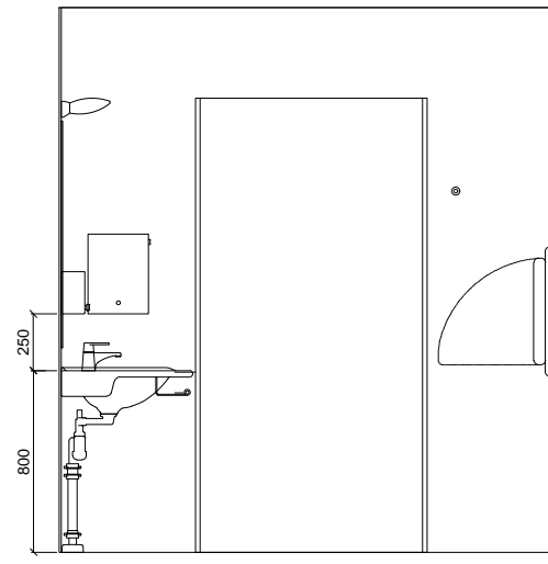
SEINÄKAAVIO F
