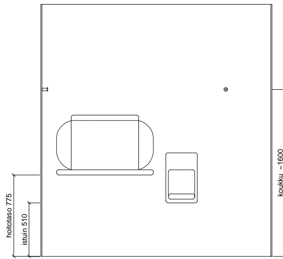
SEINÄKAAVIO G
