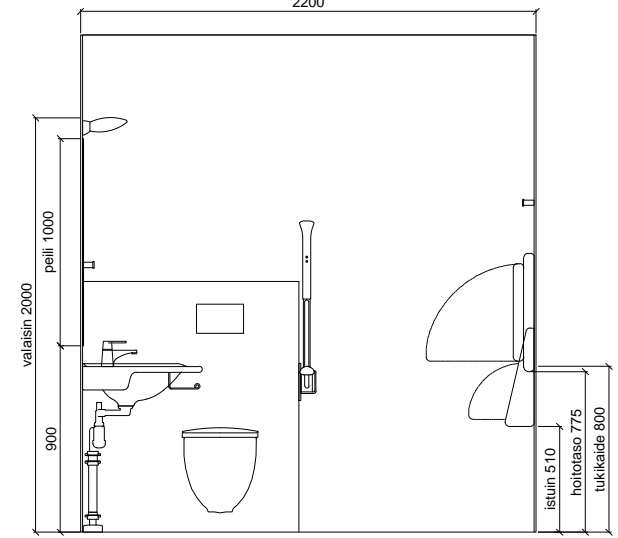
SEINÄKAAVIO D
