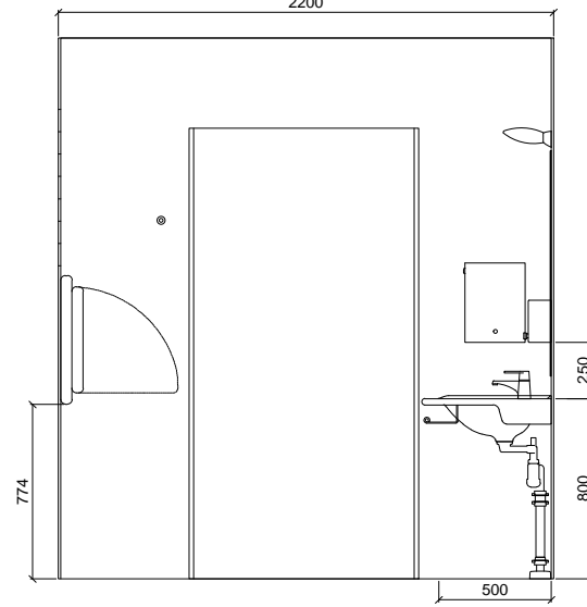
SEINÄKAAVIO B
