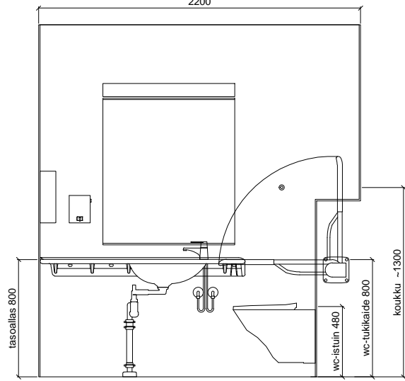
SEINÄKAAVIO A
