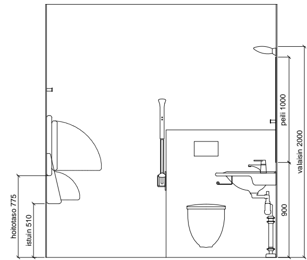
SEINÄKAAVIO H
