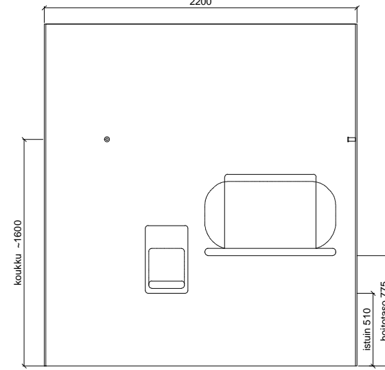
SEINÄKAAVIO C
