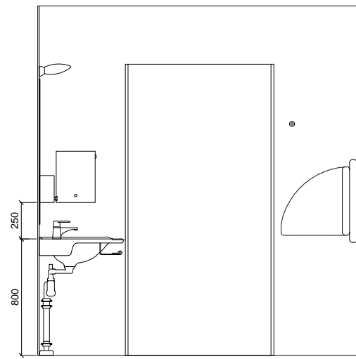
SEINÄKAAVIO F
