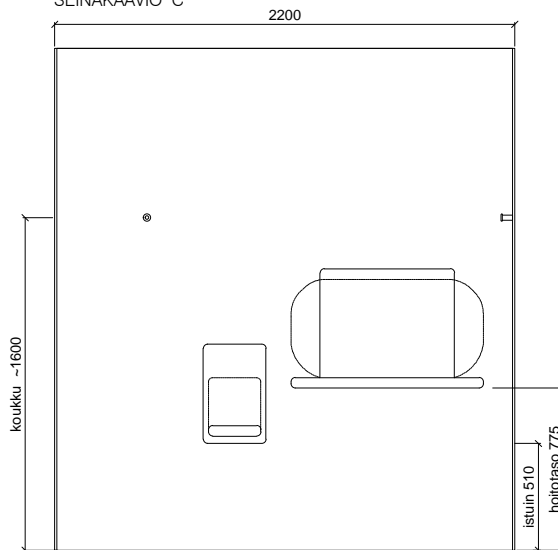
SEINÄKAAVIO C
