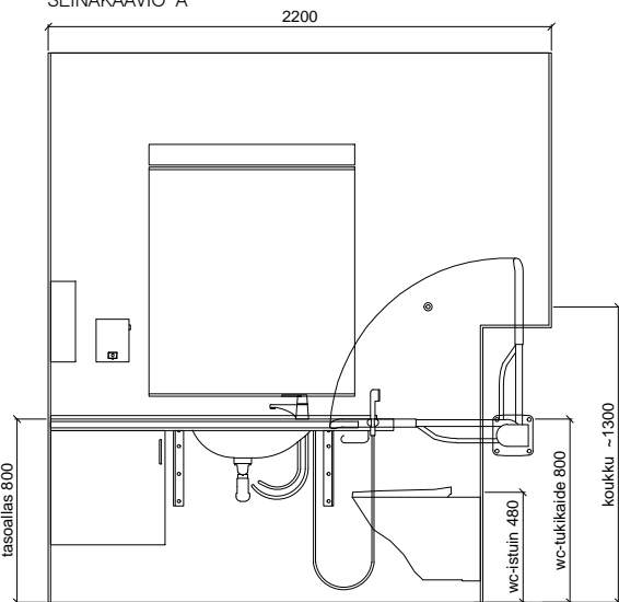
SEINÄKAAVIO A
