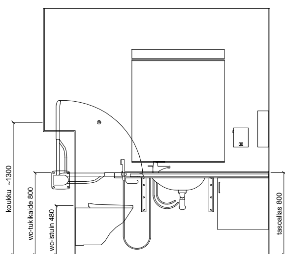
SEINÄKAAVIO E
