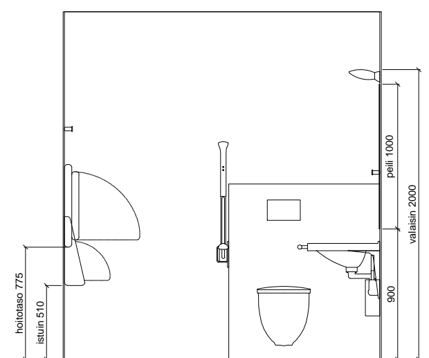
SEINÄKAAVIO H
