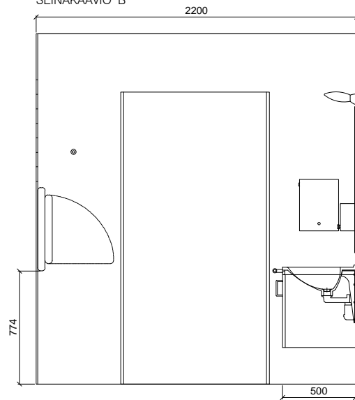
SEINÄKAAVIO B
