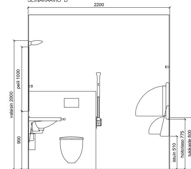
SEINÄKAAVIO D
