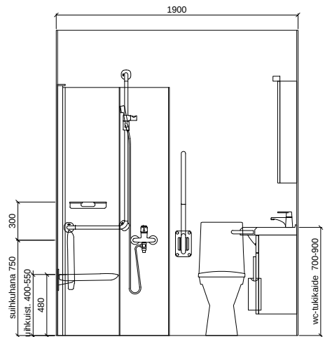
SEINÄKAAVIO D Senior
