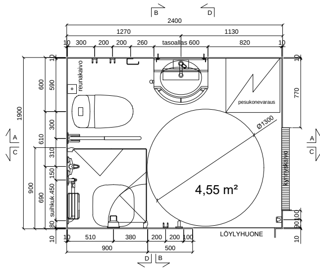
POHJAPIIRROS Senior
