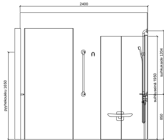
SEINÄKAAVIO C Senior
