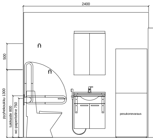
SEINÄKAAVIO A Senior
