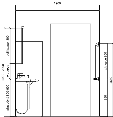
SEINÄKAAVIO B Senior
