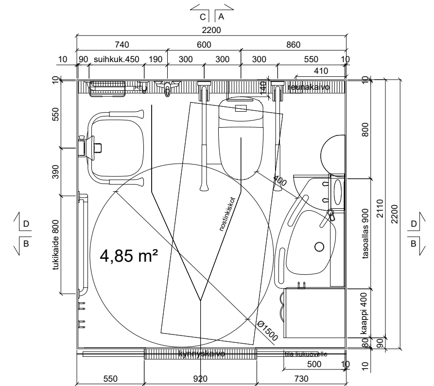
POHJAPIIRROS Gaius Sense Basin 2XL
