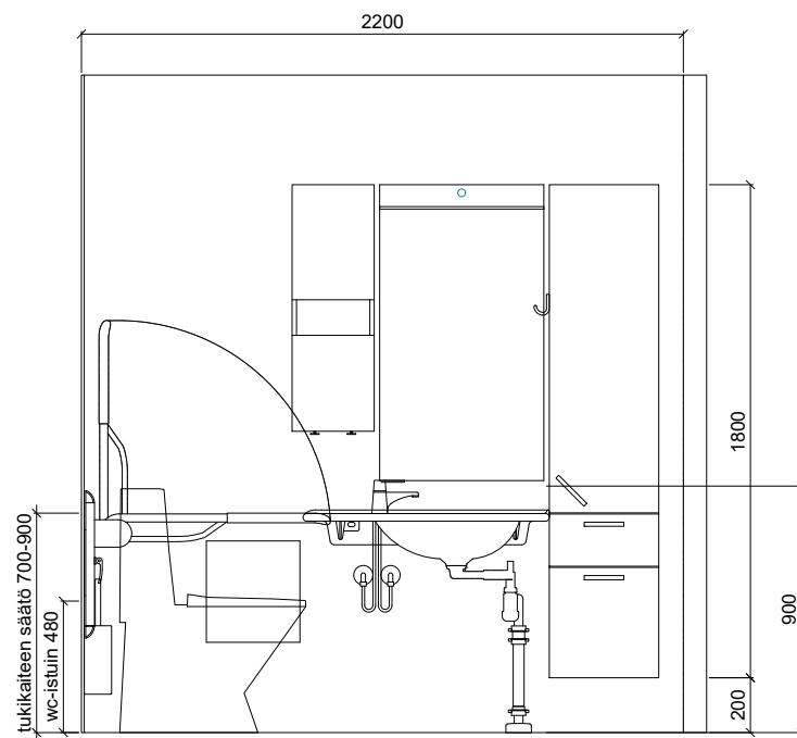
SEINÄKAAVIO A Gaius Sense Basin 2XL
