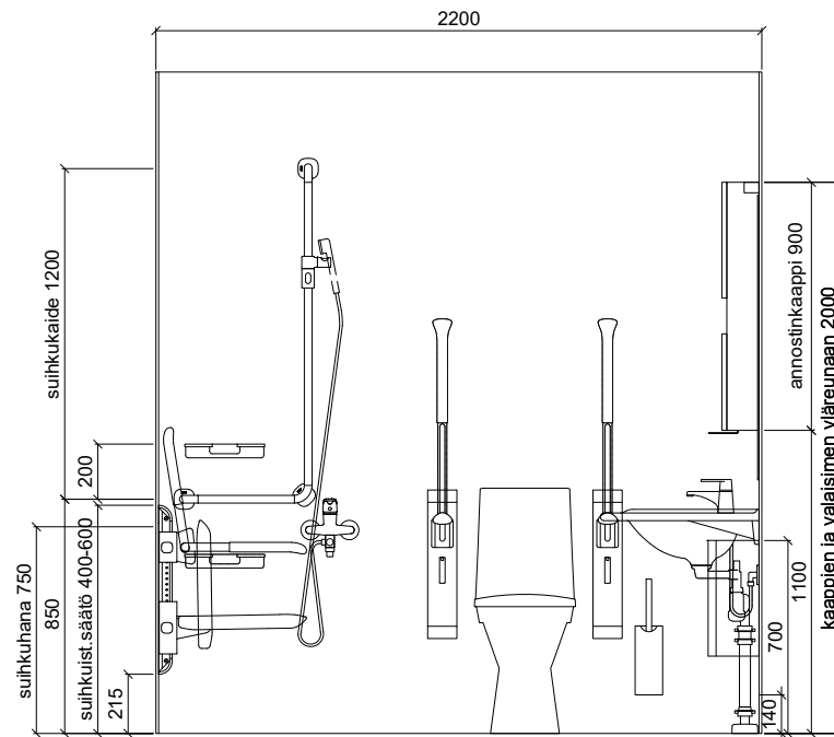
SEINÄKAAVIO D Gaius Sense Basin 2XL
