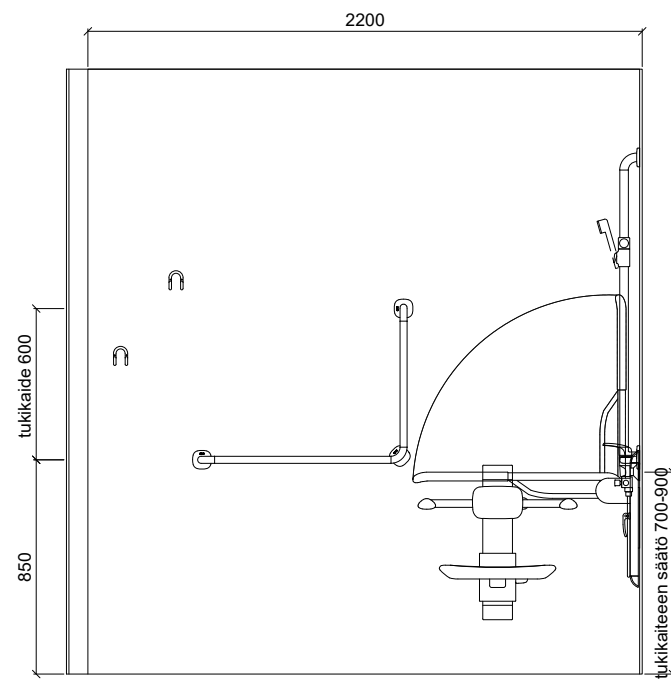
SEINÄKAAVIO C Gaius Sense Basin 2XL
