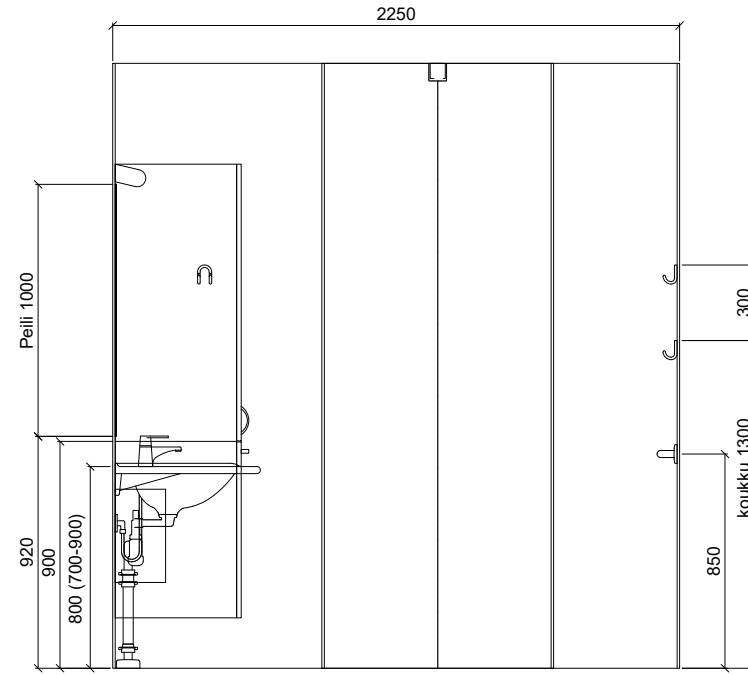
SEINÄKAAVIO B Gaius Sense Basin 3XL
