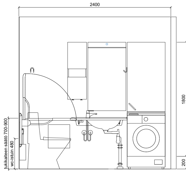
SEINÄKAAVIO A Gaius Sense Basin 3XL
