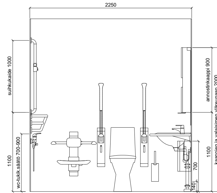
SEINÄKAAVIO D Gaius Sense Basin 3XL
