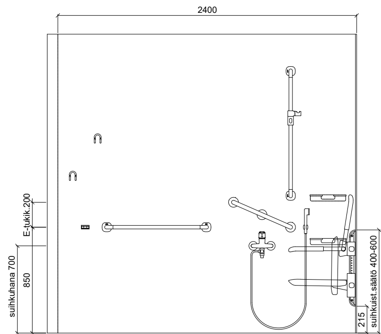
SEINÄKAAVIO C Gaius Sense Basin 3XL
