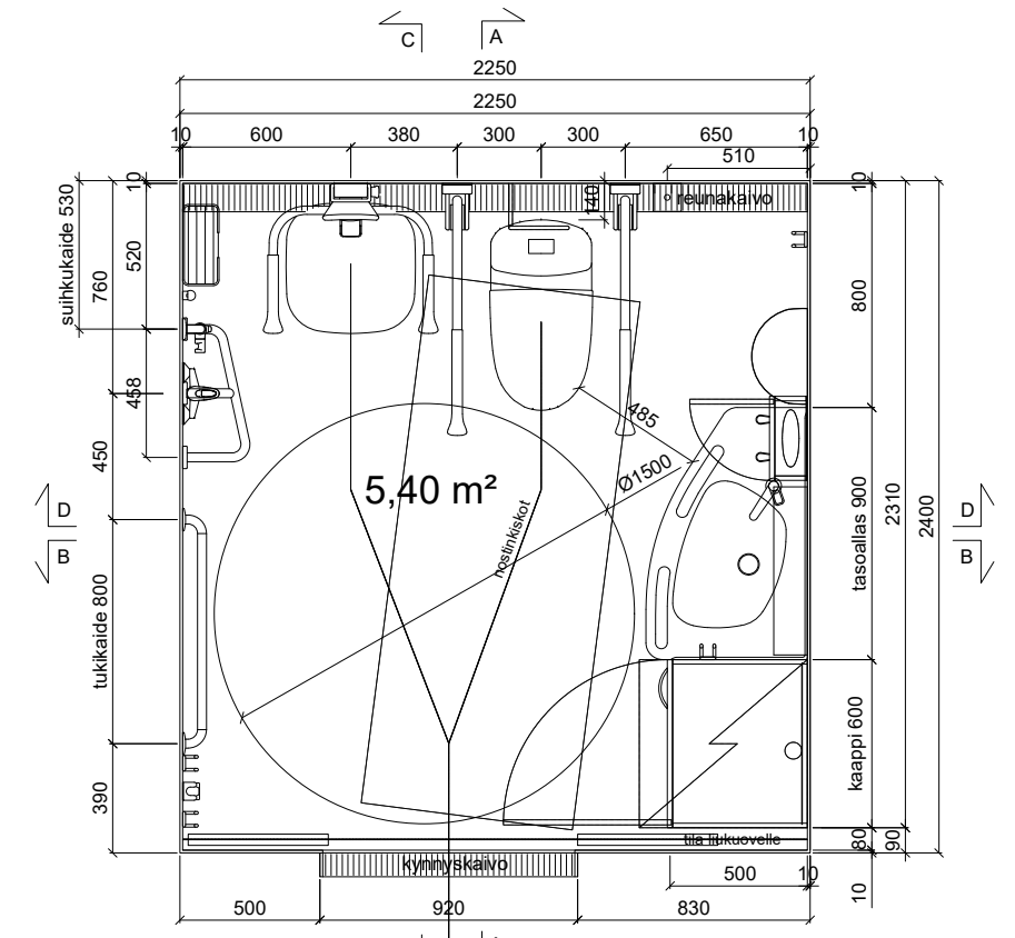
POHJAPIIRROS Gaius Sense Basin 3XL
