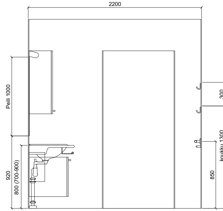
SEINÄKAAVIO B Gaius Sense Plus 1500
