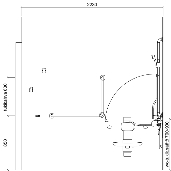
SEINÄKAAVIO C Gaius Sense Plus 1500
