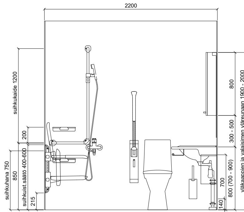
SEINÄKAAVIO D Gaius Sense Plus 1500
