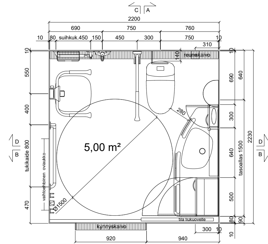
POHJAPIIRROS Gaius Sense Plus 1500
