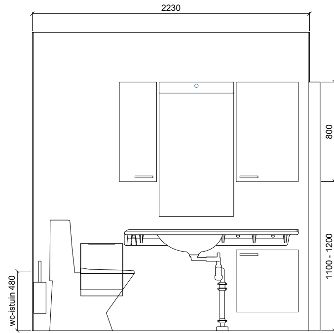
SEINÄKAAVIO A Gaius Sense Plus 1500
