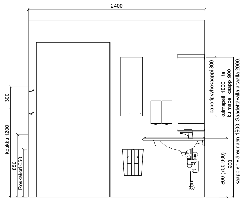
SEINÄKAAVIO A Gaius Hospital Sense XL, DUO
