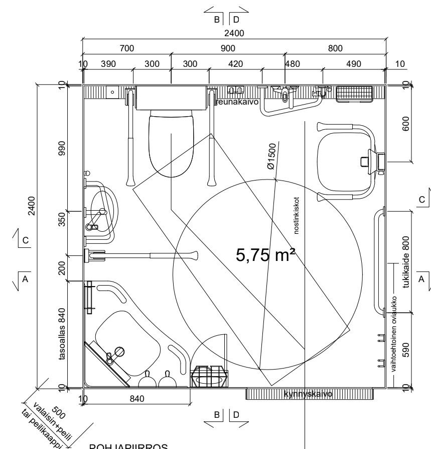
POHJAPIIRROS Gaius Hospital Sense XL, DUO
