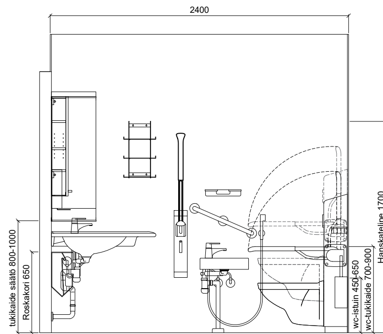
SEINÄKAAVIO B Gaius Hospital Sense XL, DUO
