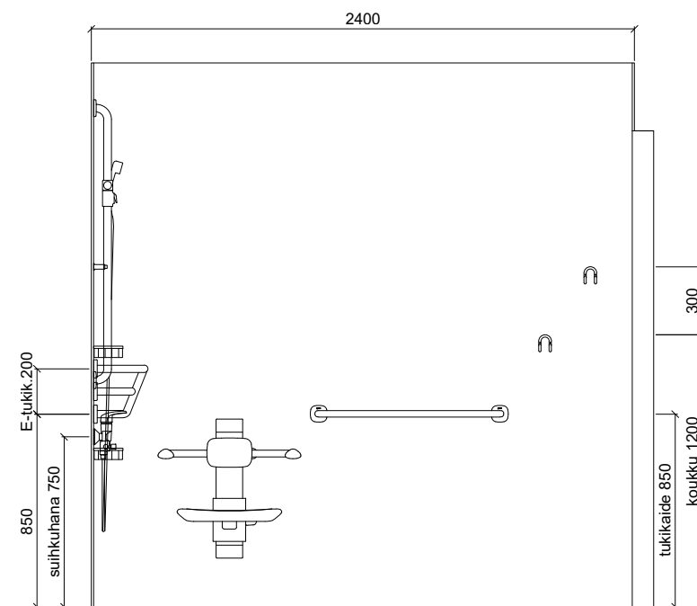
SEINÄKAAVIO B Gaius Hospital Sense XL, DUO
