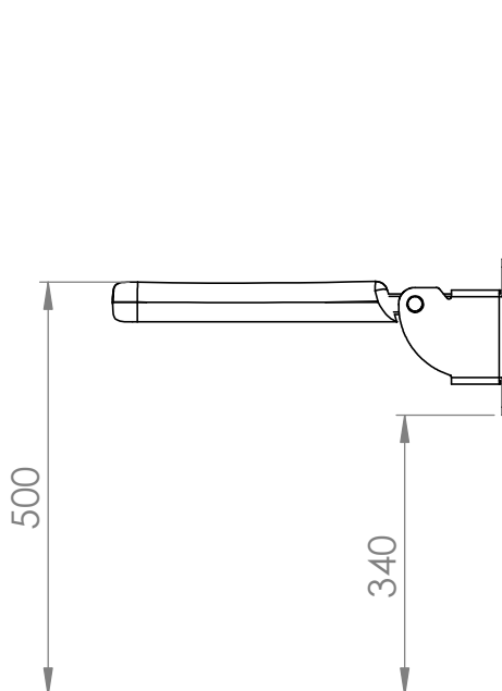
Kiinteät suihkuistuimet Fixed shower seats
