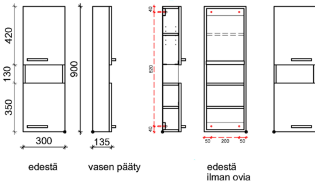
pystyleikkaus
